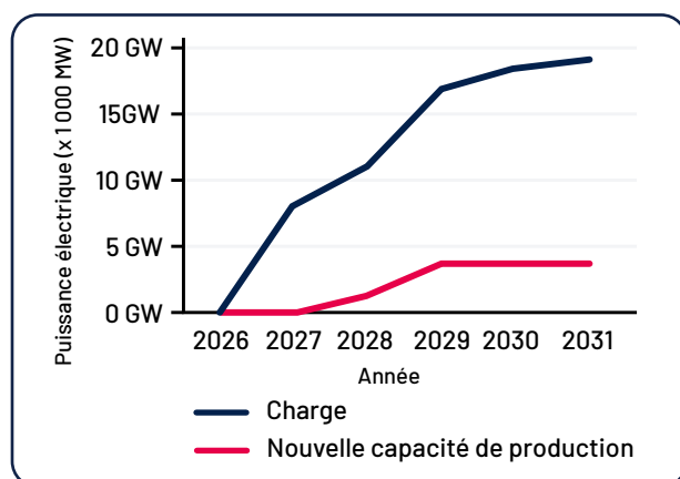
Figure 4. Charge des centres de données en Alberta par rapport aux nouvelles capacités de production
